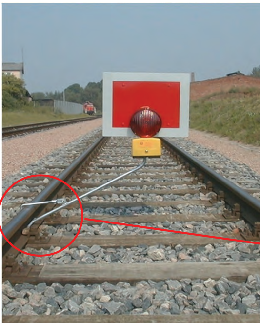
Signal Sh 2, mit Klemmständer und EBA zugelassener Signalleuchte
