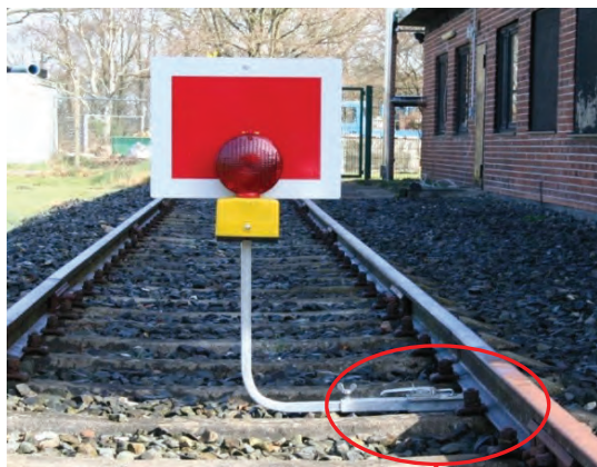
Signal Sh 2, mit mit Klappständer abschliessbar in beiden Lagen durch handelsübliches Vorhängeschloss
